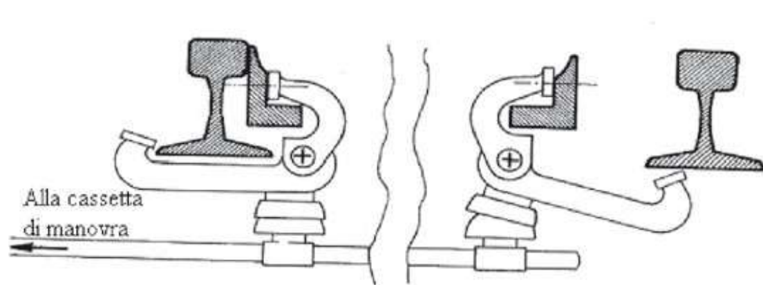
Schema del movimento dello scambio
