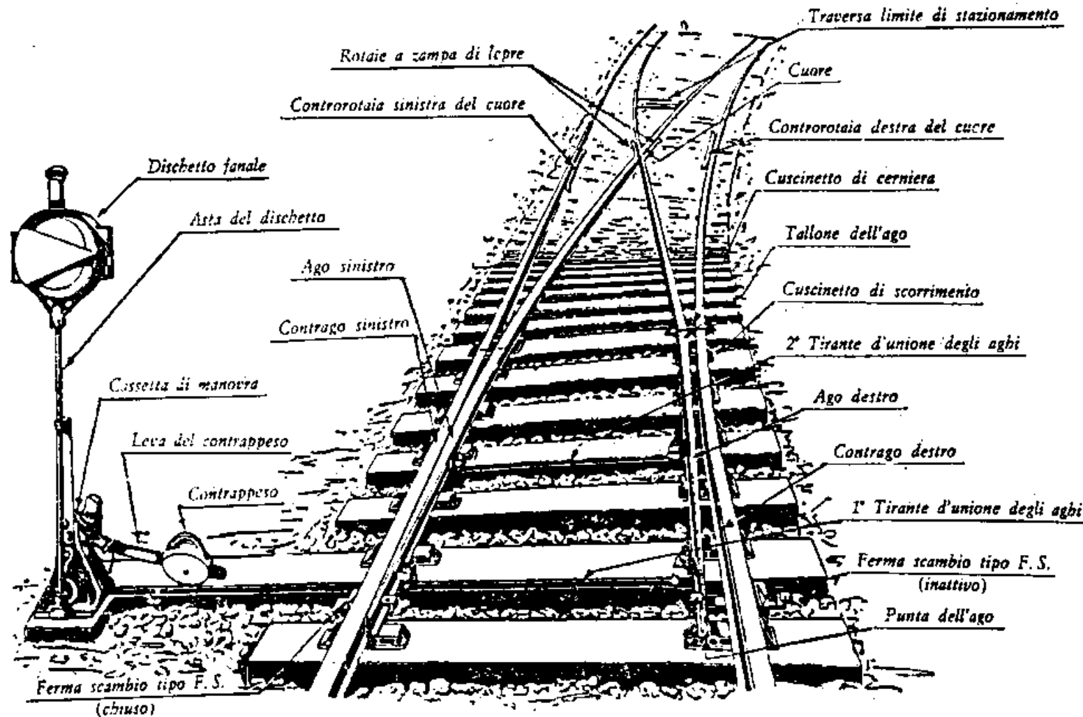
- Parti di un deviatoio semplice (nomenclatura)
